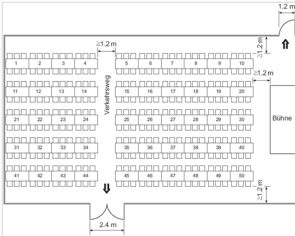
Bild 3: Beispiel einer Bankettbestuhlung mit den notwendigen Fluchtwegen.
