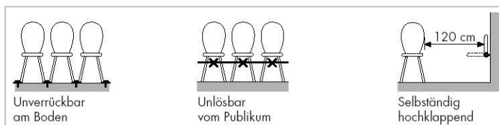
Bild 2: Befestigung der Bestuhlung.
